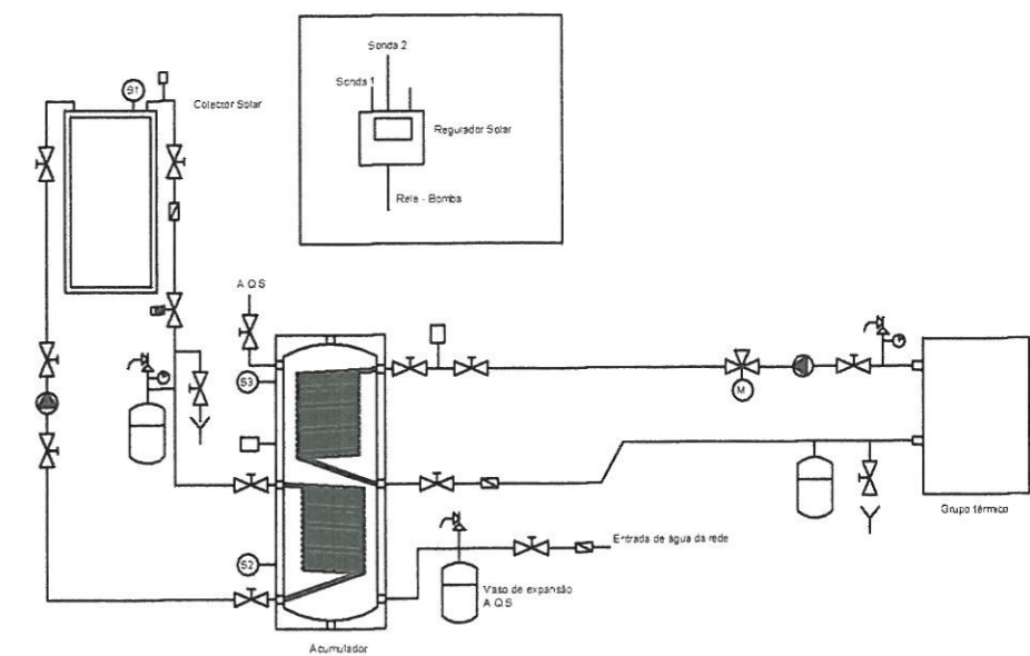
Esquema do Grupo SolarTérmico
